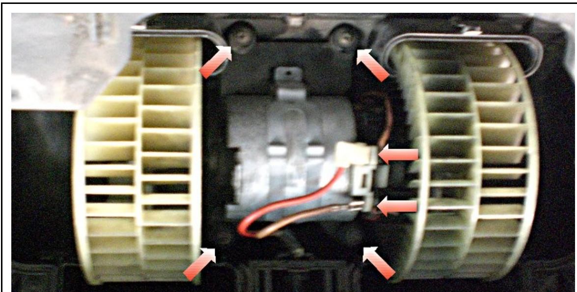
Abbildung 10: Der Gebläselüfter liegt nun frei. Zum Ausbau des Gebläsemotors sind die beiden Anschlusskabel zu lösen und die vier Kreuzschlitzschrauben zu entfernen. Danach kann der Gebläsemotor mitsamt seiner Halterung heraus gehoben werden.
