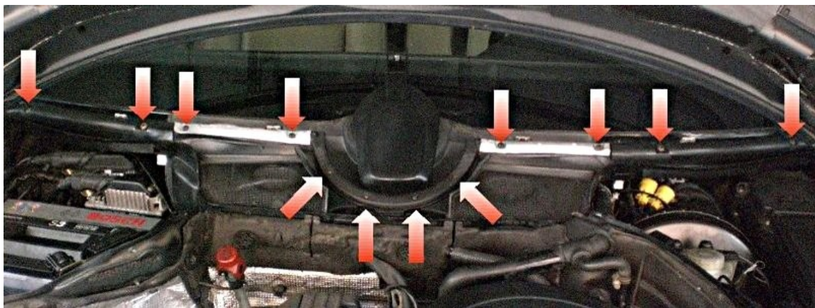
Abbildung 4: Alle Schrauben am Windschutzscheibenrahmen rechts und links des Scheibenwischers und rund um den Scheibenwischer entfernen. Die äußeren Schrauben sind kürzer als die zum Wischer hin gewandten. Am Besten ist es, wenn die Schrauben nach Entfernen der Abdeckungen wieder an ihren ursprünglichen Platz leicht eingeschraubt werden.
