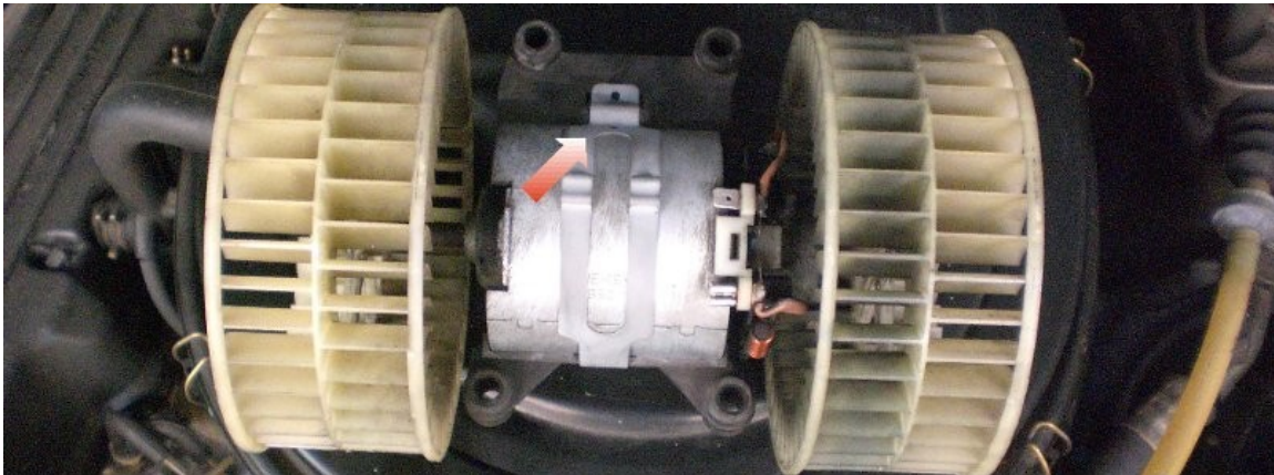
Abbildung 12: Der Gebläselüfter wird durch eine starke Klammer im Sockel gehalten.
